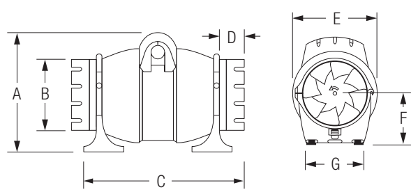
ELLP125
