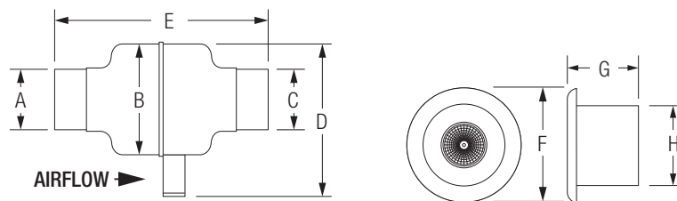
EL100
