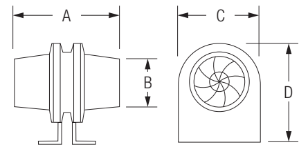
ELLP150 / EL150
